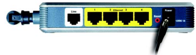
Figure 4-5 : Connexion de l'alimentation
